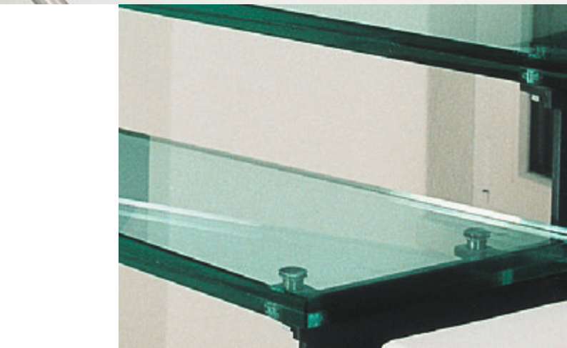
Aufgesattelte Metallwangentreppe mit Glasstufen. Geländer mit T-Pfosten, INOX-Seilen und CNS-Handlauf.
